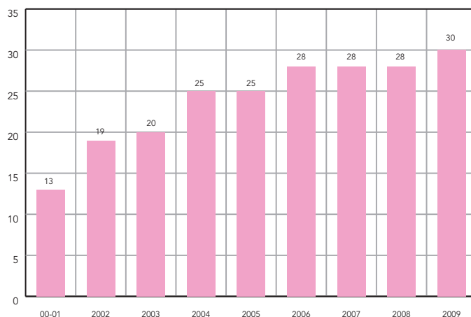
Cadro 73 Evolución do número de proxectos e convenios no CITEEC
