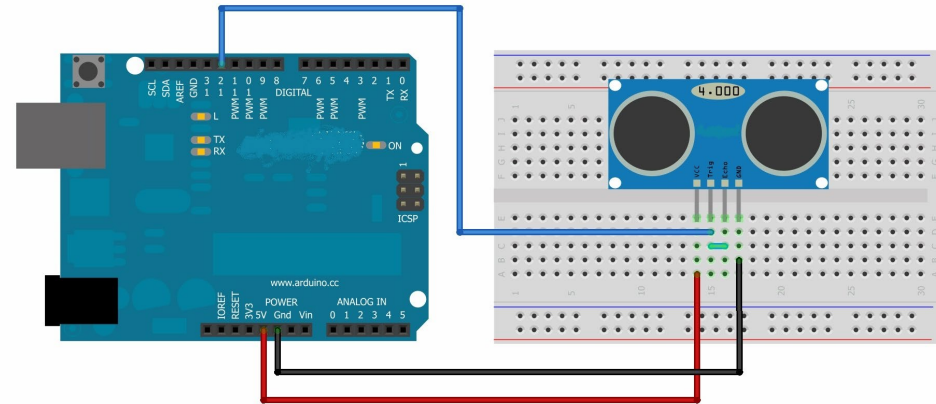
Figura 1. Circuito Arduino. Fuente: lahmed2, Arduino circuit . Licencia CC-BY-SA-3.0
